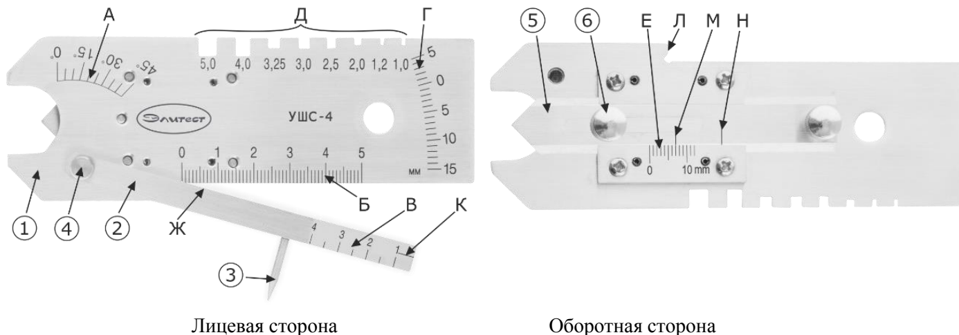
Рисунок 1 – Общий вид универсального шаблона сварщика УШС-4 ЭЛИТЕСТ
