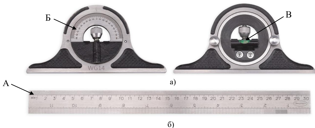
Рисунок 1 – Общий вид измерительного шаблона сварщика WG14 ЭЛИТЕСТ
